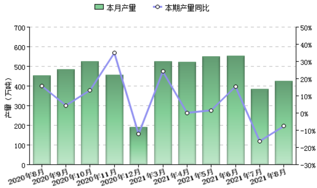
2021年8月陕西省水泥熟料产量和同比增长率
