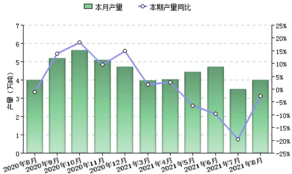
陕西省2021年8月隔热保温材料本月产量和同比增长率
