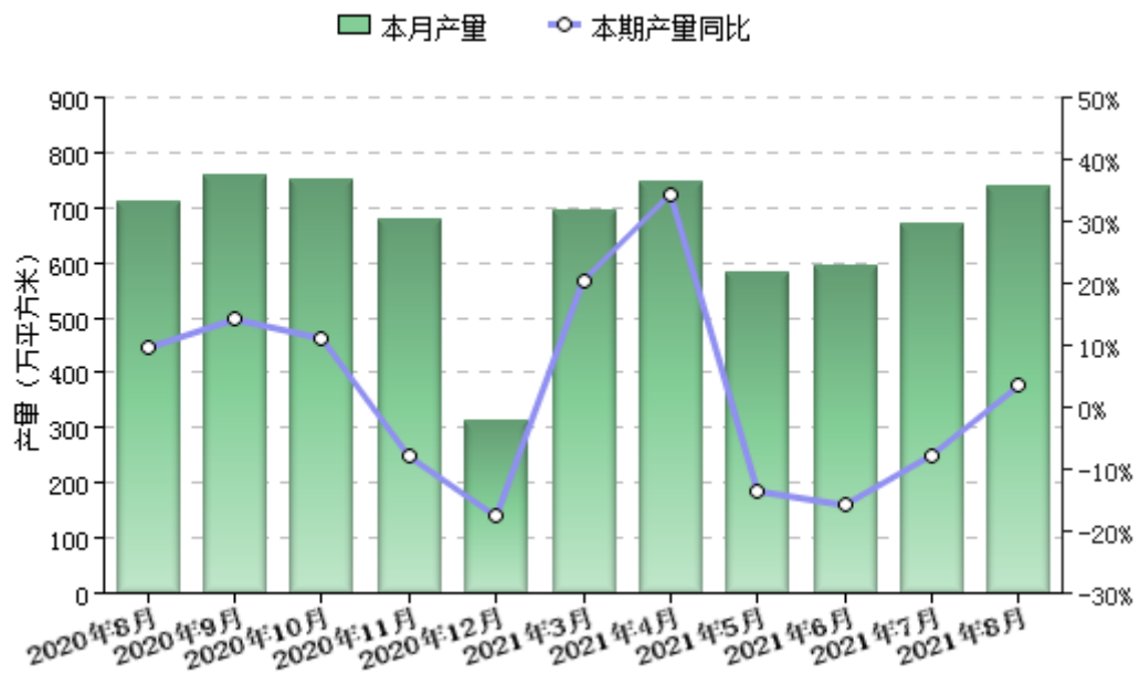
2021年8月陕西省石膏板产量和同比增长率
