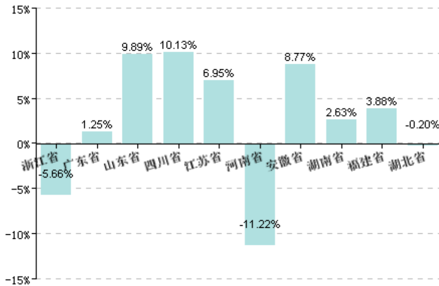
2021年8月商品混凝土周边地区同比增长率
