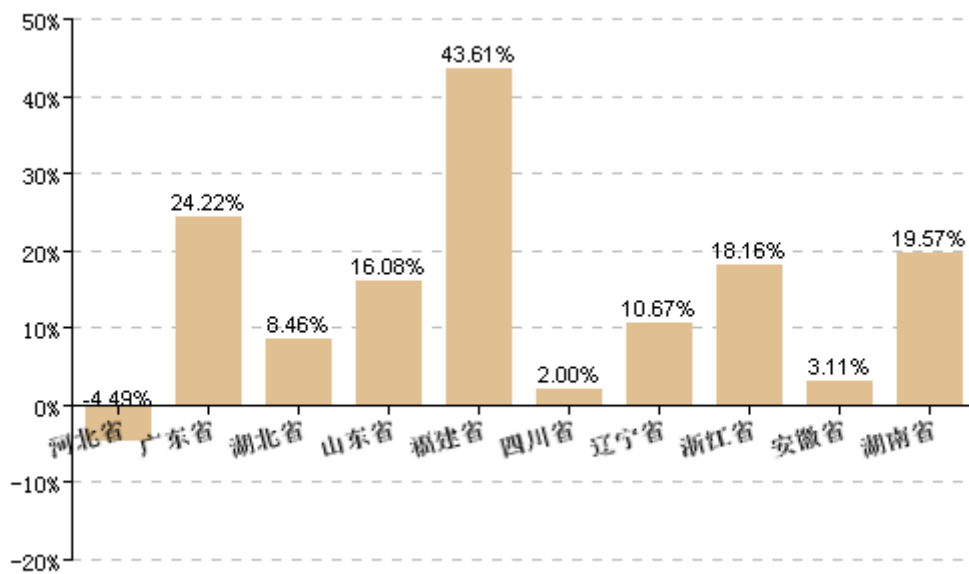
2021年8月平板玻璃周边地区累计同比增长率
