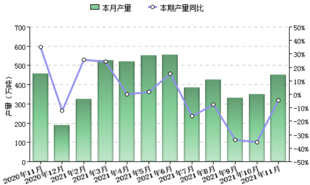
2021年11月陕西省水泥熟料产量和同比增长率
