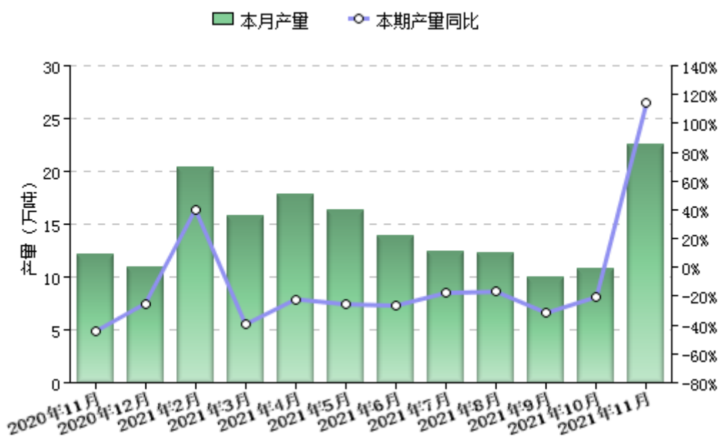
2021年11月陕西省石灰产量和同比增长率
